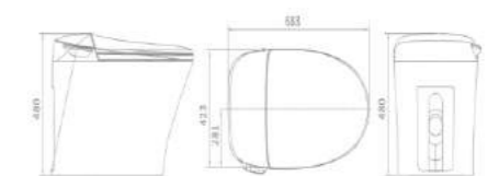
TKM-132 Size : 683x423x480mm S-trap : 300/305mm
